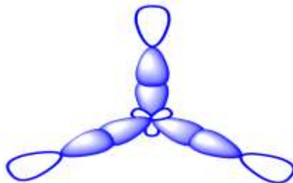
Sự hình thành phân tử \text{BF}_3
