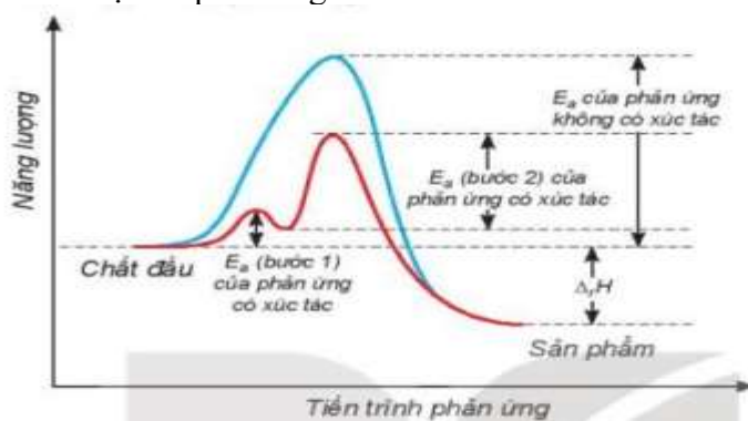
Hình 3.1. Ảnh hưởng của xúc tác đến năng lượng hoạt hóa
