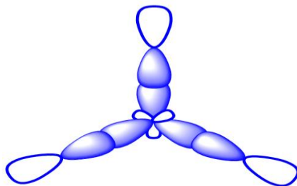
Sự hình thành phân tử \text{BF}_3
