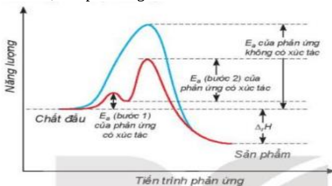
Hình 3.1. Ảnh hưởng của xúc tác đến năng lượng hoạt hóa
