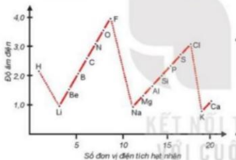
Hình 6.4. Sự biến đổi độ âm điện theo chu kỳ và nhóm
