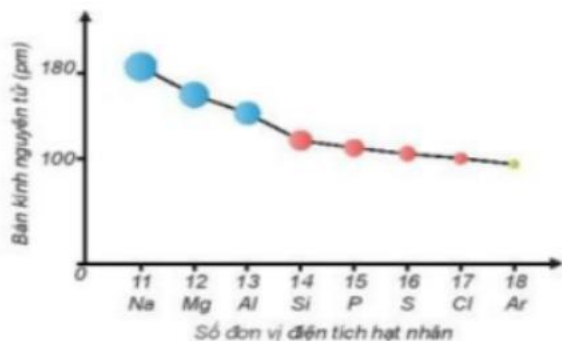
Hình 6.1. Sự giảm bán kính nguyên tử của các nguyên tố trong chu kỳ 3
