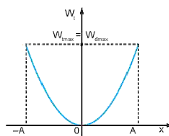
Hình 5.2. Sự biến thiên của thế năng W_t theo li độ x
