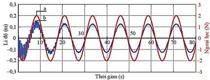
Hình 6.3. Thí nghiệm về dao động cưỡng bức
