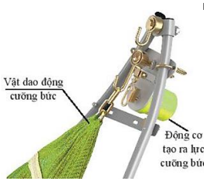
Hình 4.7. Vồng máy tự động sử dụng điện
