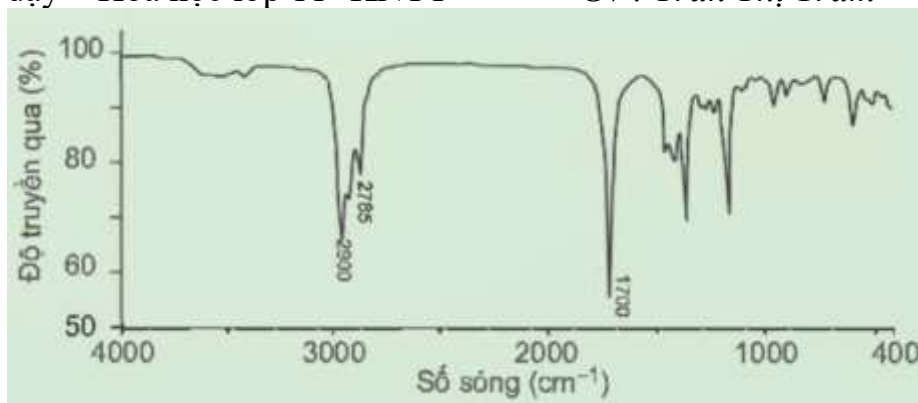
Bảng 10.2. Số sóng hấp thụ đặc trưng trên phổ hồng ngoại của một số nhóm chức cơ bản
