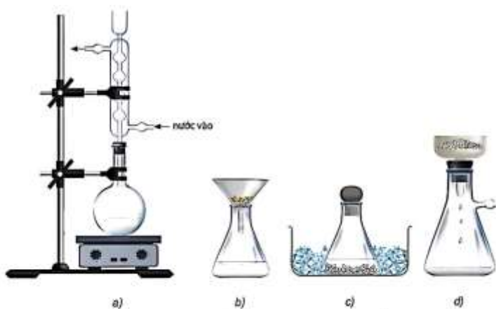
Hình 11.7. Các bước tiến hành trong phương pháp kết tinh
