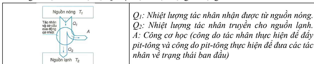
Hình 2.6 a) Sơ đồ nguyên tắc hoạt động của động cơ nhiệt
