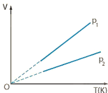
Hình 10.2. Các đường đẳng áp
